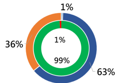
氣冷式能效等級
